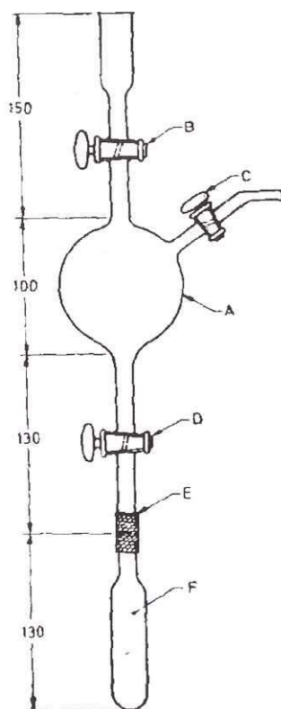
FIG. 1 NAKAZONO REDUCTOR
